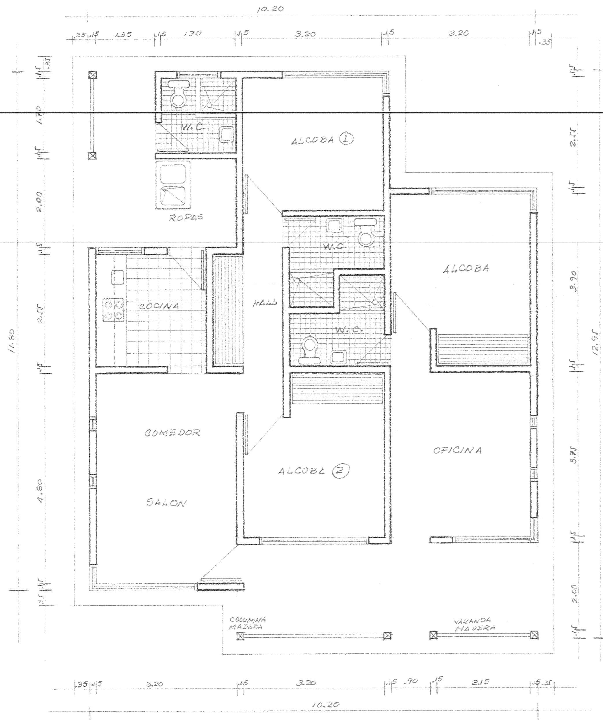
PLANTA GENERAL ESC: 1:50
